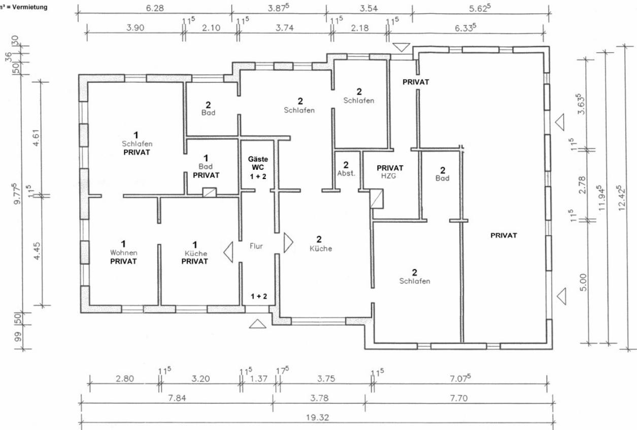
Grundriss
